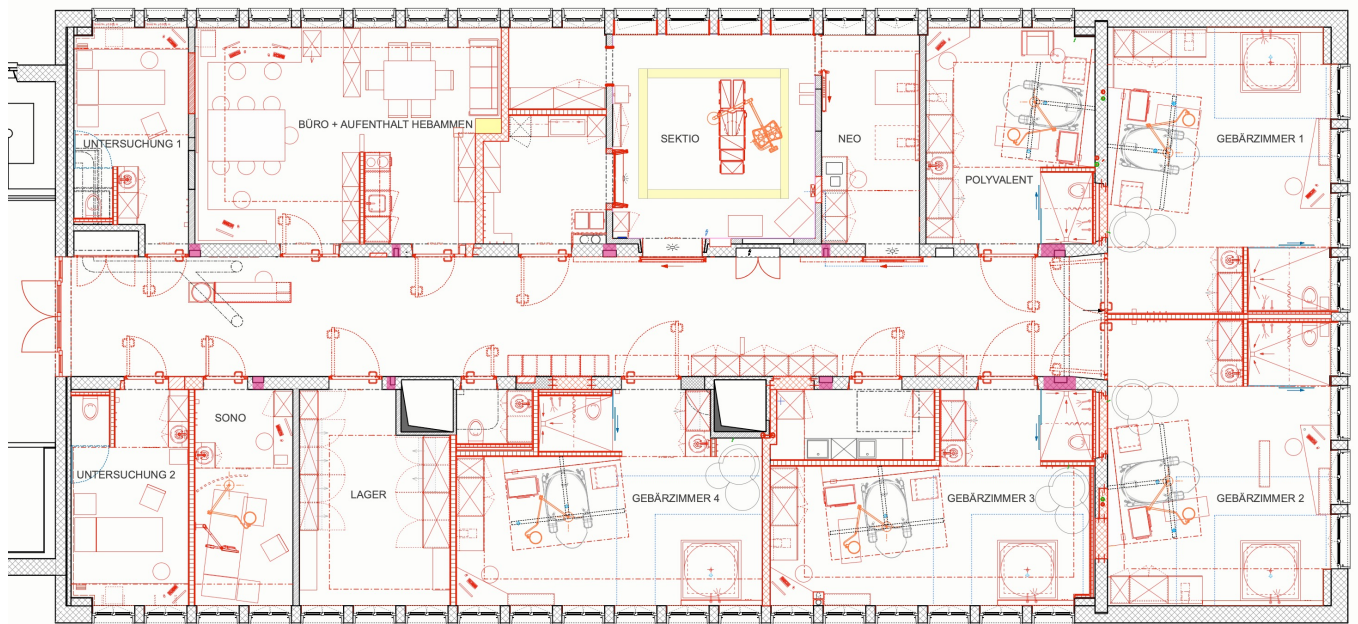
Grundriss 3. Obergeschoss
